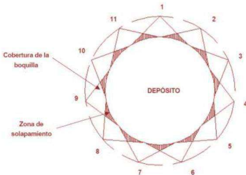
Ilustración 33 Distribución y solapamiento de las boquillas
