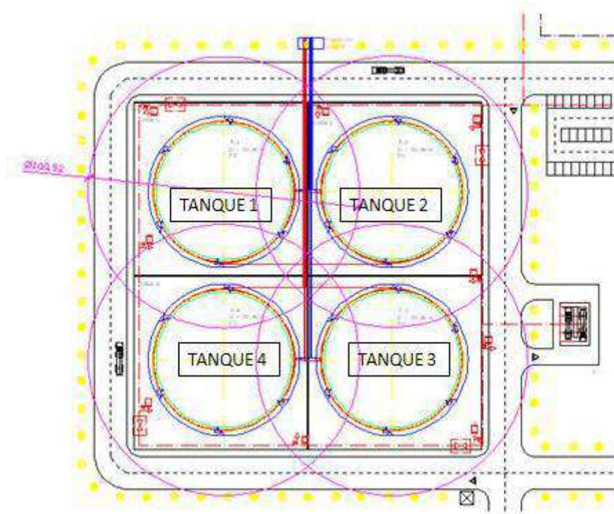
Ilustración 12 Tanques afectados por la radiación
