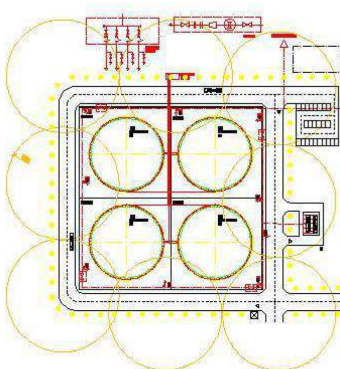
Ilustración 13 Distancia de cualquier punto de la planta a un hidrante
