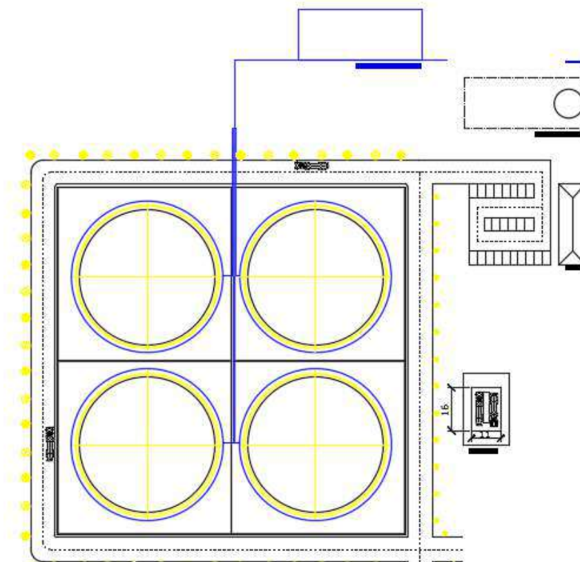
Ilustración 16 Esquema del sistema de espuma
