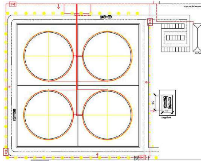
Ilustración 10 Implantación de tuberías de agua.
